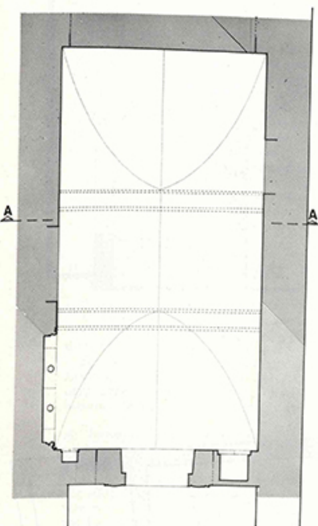
ΣΧΕΔΙΟ 2 ΚΑΤΩΨΗ
