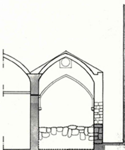
TOMH B-B
